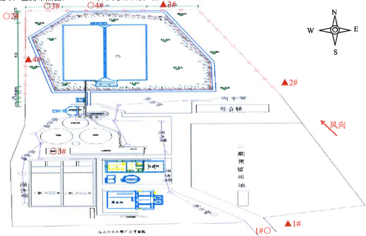
附图 1: 检测布点图, “○”表示无组织废气检测点; “▲”表示厂界噪声检测点
